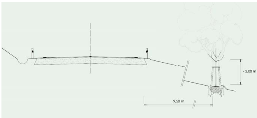
U komunikace v násypu 2 m nad terénem je potřeba sadit stromy minimálně 9,5 m od vozovky
