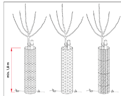
Ochrana kmene při jednobodovém kotvení: drátěné pletivo, plast, rákos apod. (Příloha č. 5 standardy SPPK-C02-03)
