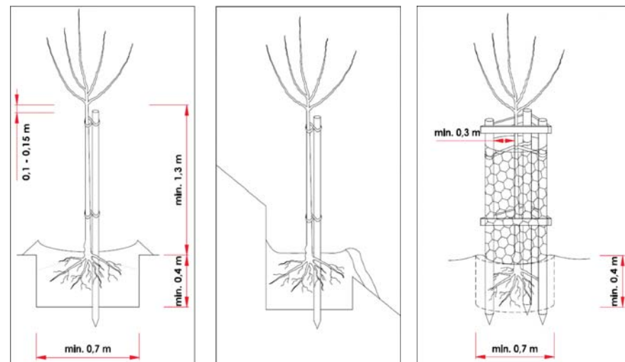
Výsadba ovocného stromu na rovině/na svahu (Příloha č. 5 standardy SPPK-C02-03)
